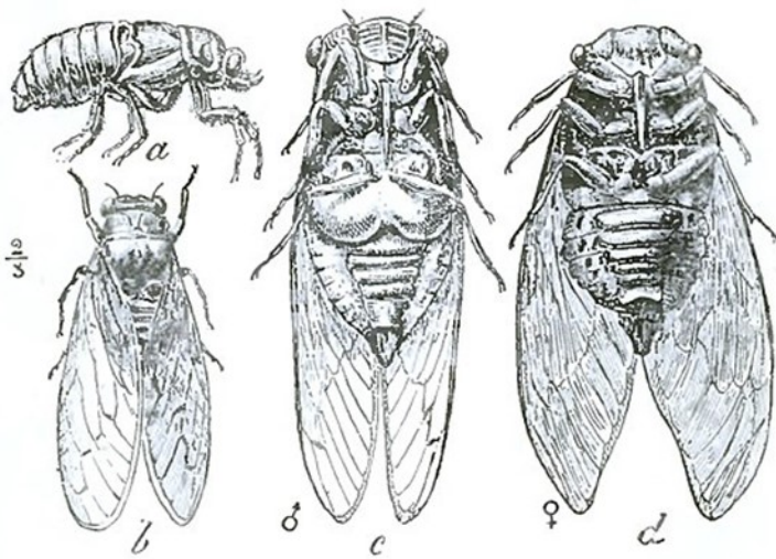
Cycle de vie de la cigale
